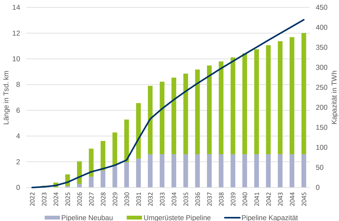
Abbildung 8: Wasserstoff-Pipelinenetz: Länge (in Tsd. km) und Kapazität (in TWh)
