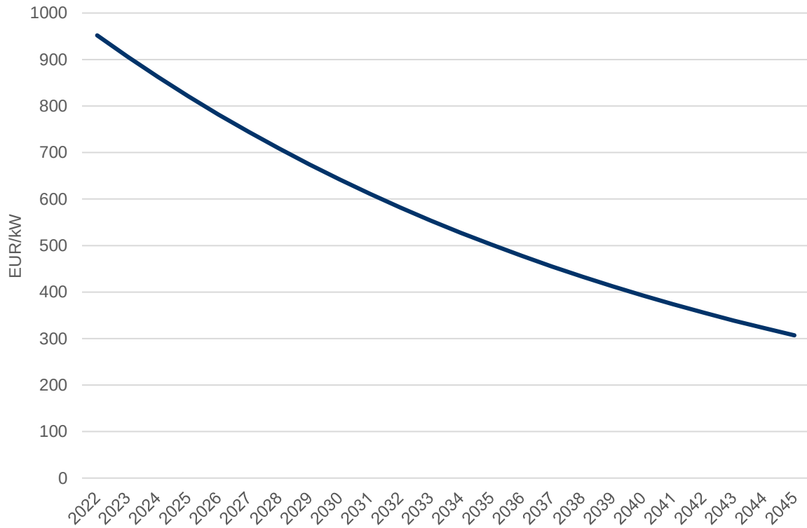
Abbildung 23: Investitionskosten für Elektrolyseure (in EUR/kW)
