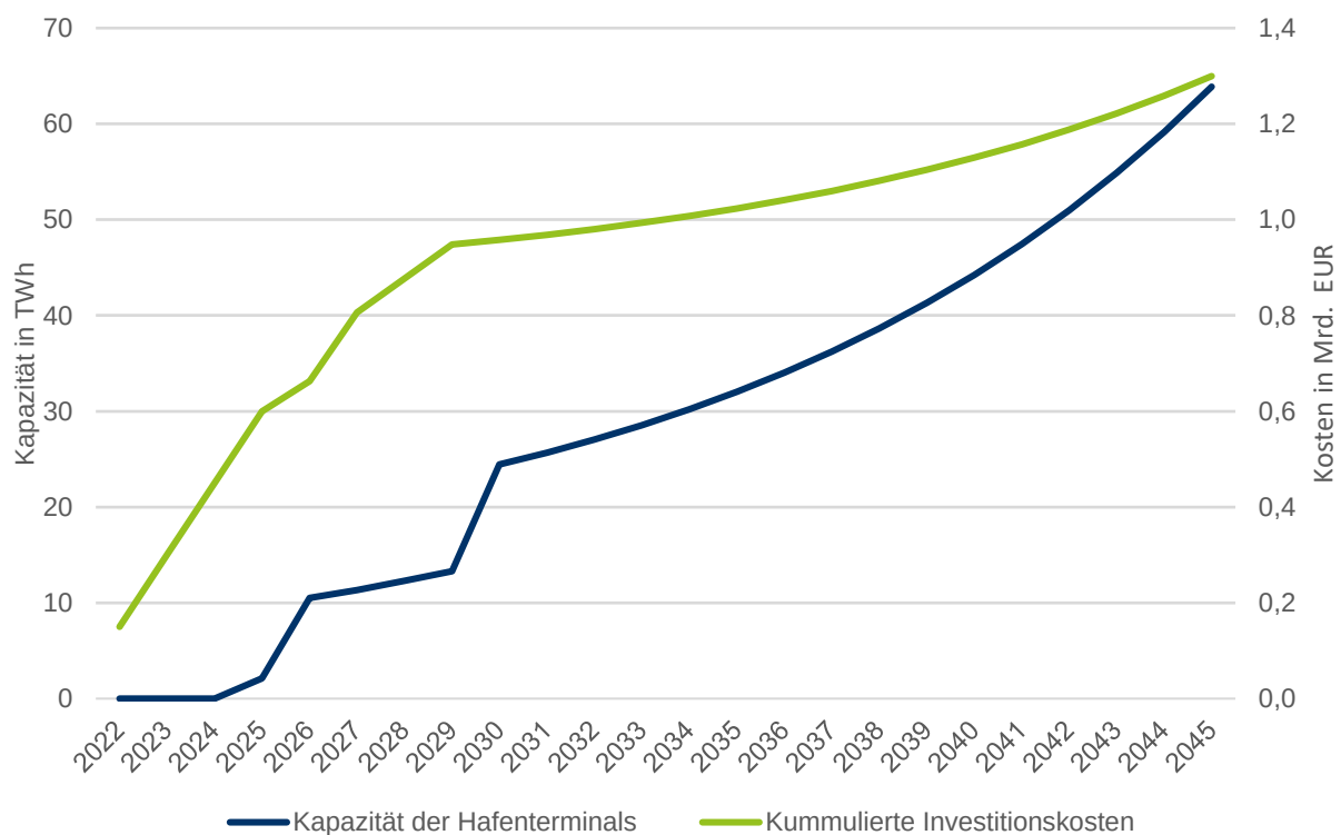
Abbildung 6: Kapazität (in TWh) und Investitionskosten (in Mrd. EUR) der Häfen
