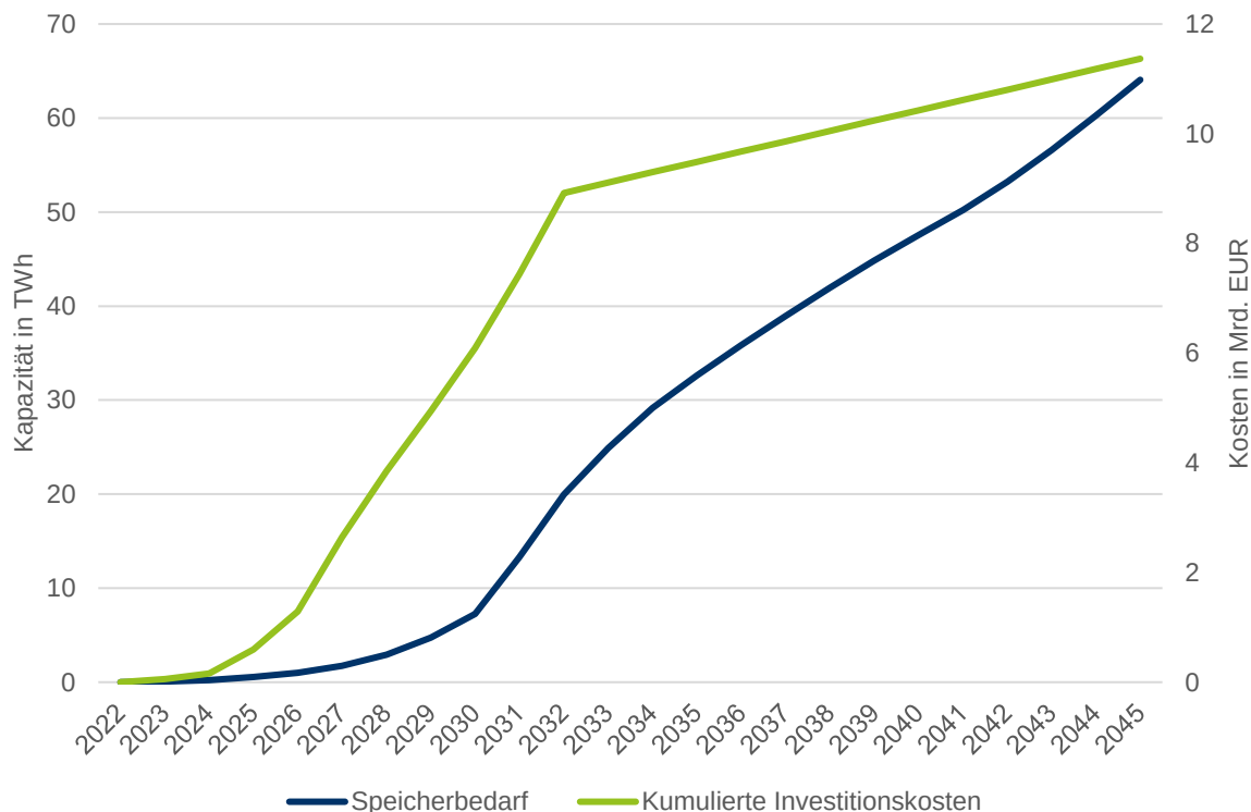
Abbildung 7: Wasserstoff-Speicherbedarf (in TWh) und Investitionskosten (in Mrd. EUR)
