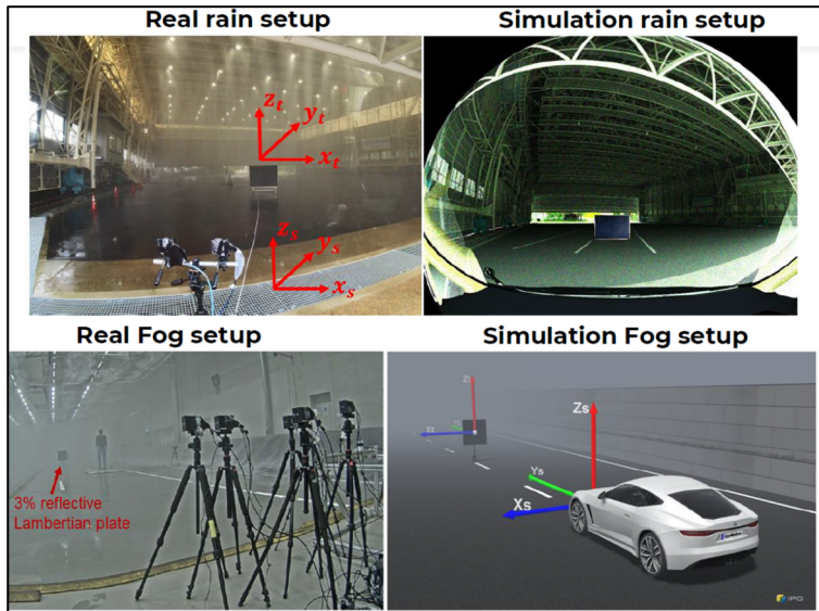
Abbildung: Reale und virtuelle Testumgebungen für Untersuchung des einflusses von Regen und nebe. (Quelle: https://doi.org/10.3390/s23156891 )
